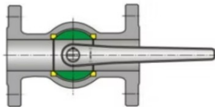
'ON' Position
